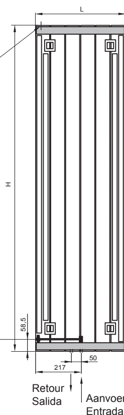
Achteraanzicht ventielradiator Vista trasera radiator con válvula integrada
